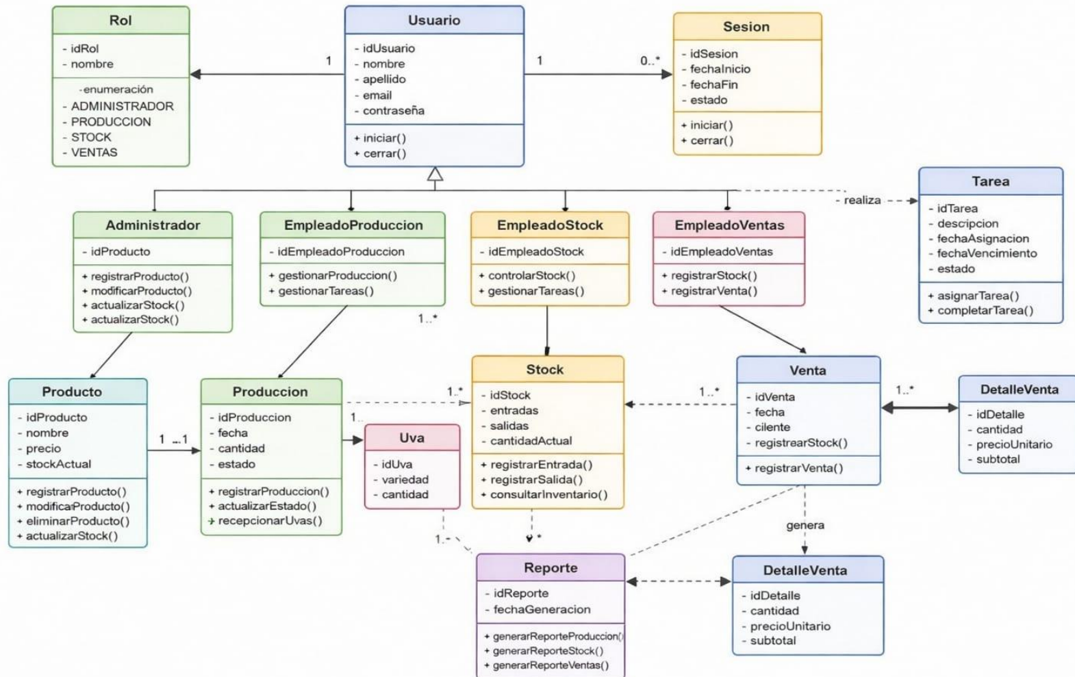
DIAGRAMA UML DE CLASES - SISTEMA DE GESTIÓN DE BODEGA
